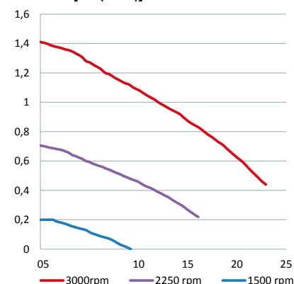
Curva H/Q [Bar(m 3 /h)]
