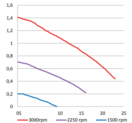
Curva H/Q [Bar(m 3 /h)]
